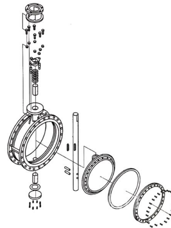
三偏心蝶阀的结构爆炸图
