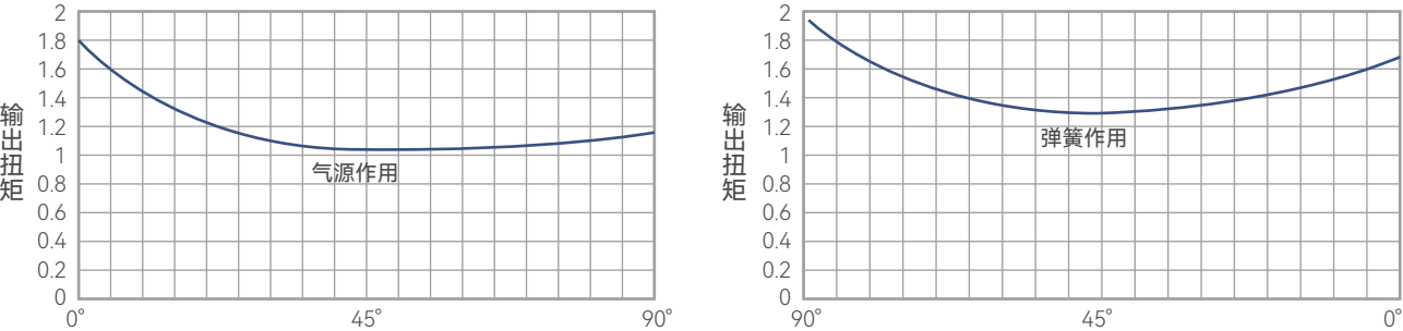
单作用执行器扭矩表
