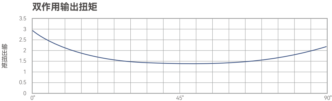
双作用执行器扭矩表
